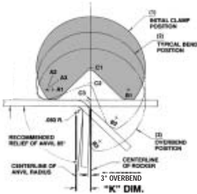
Bender Location ... "K" Dim.
